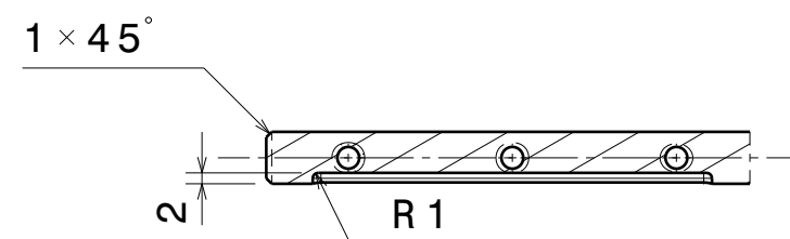
SECCION A-A ESCALA: 2:3
